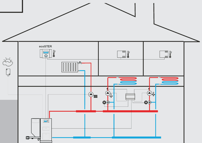
Rys 2 - ecoSTER 200 z dwoma dodatkowymi czujnikami pokojowymi
