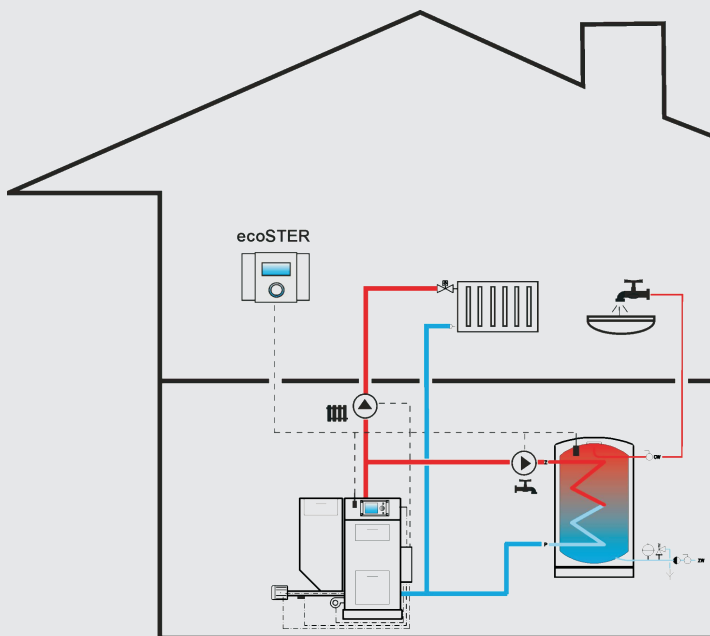
Rys 1 - ecoSTER 200 (wbudowany czujnik temperatury)
