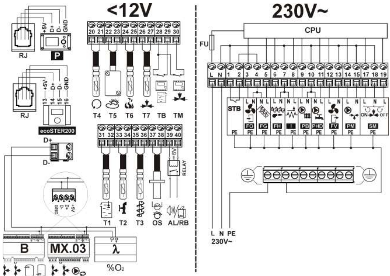
Мал. 22 Схема електричних з'єднань контролера, де: T1-датчик температури котла СТ4, T2-датчик температури гарячої води СТ4, T3-датчик температури подачі, OS-оптичний датчик полум'я, AL/RB-місце підключення сигналу зовнішньої тривоги або резервного котла, RELAY-контактор, T4-датчик температура повернення СТ4, T5-зовнішній датчик температури СТ4-Р, T6-датчик температури парів СТ2S, T7-датчик температури змішувача, ТВ-місце підключення термостату котла, ТМ-місце підключення термостату змішувача, Р-панель керування, есоSTER200-кімнатна панель з функцією кімнатного термостата (заміна ТВ або ТМ), D-D+ - підключення додаткових модулів, В-модуль В дозволяє обслуговувати ще два змішувача і буфер опалення, МХ.03 - додатковий модуль дозволяє обслуговувати два додаткових змішувачів та циркуляційного насоса, λ-модуль лямбда-зонда, L N PE-електроенергія 230, FU-запобіжник, L N PE-місце підключення обмежувача температури, FO-вентилятор пальника, FG-основний шнек, FH-шнек пальника, I-запальник, PB-насос котла або буфера, PHD-насос гарячої води, FV-вентилятор витягу котла, PM-насос змішувача, SM-сервопривід змішувача, CPU-процесор.
