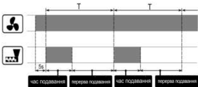
Мал. 6 Цикли роботи вентилятора і подавача
