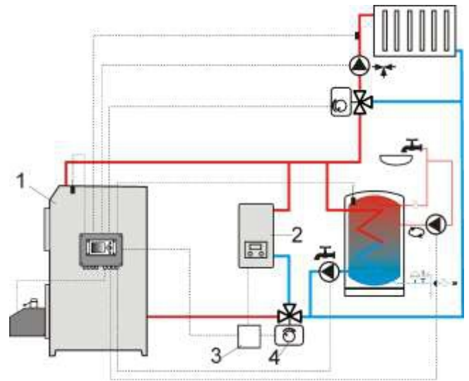
Мал. 24 6 Гідравлічна схема з додатковим котлом в замритій системі, де: 1-контролер, 2-додатковий котел, 3-контактор, 4-сервопривід клапана (з мікріками).
