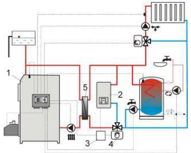
Рис. 25 липня Гідравлічна схема з додатковим котла в відкриті - замкнутий контур, де : 1 - контролер, 2 -додатковий котел, 3 - передавач, 4 - перемикання клапан (з кінця комутатори), 5 - теплообмінник,
