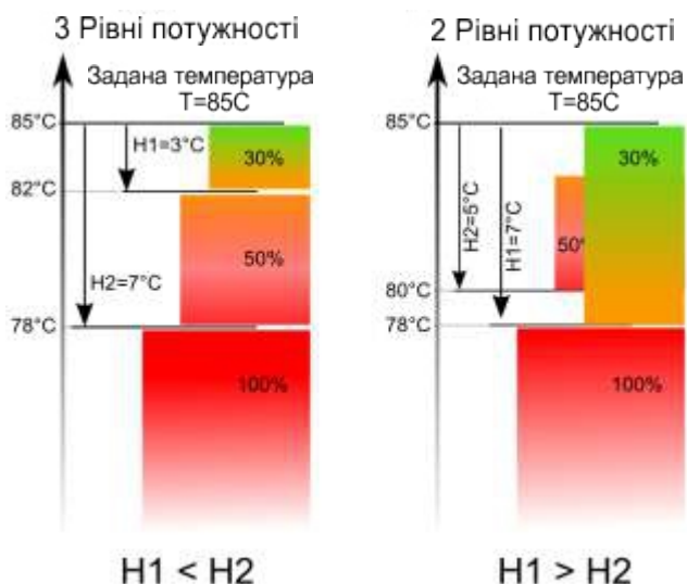
Мал. 8 Гістерезис Н1 та Н2 модуляції потужності.
