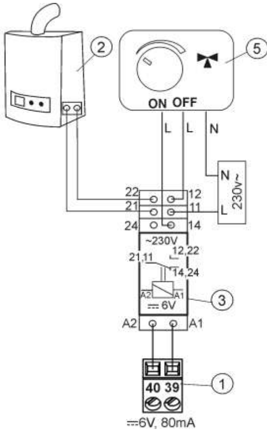
Мал. 26 Електричні схеми управління контактором додаткового котла, де: 1-контролер, 2-додатковий котел, 3-контактор, 5 - сервопривід клапана змішувача (з мікрокама), увага: клеми 22, 21, 24 повинні бути відокремлені від клем 12, 11, 14.
