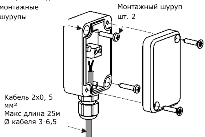
Рис. 23 Подключение датчика погоды СТ4-Р.
