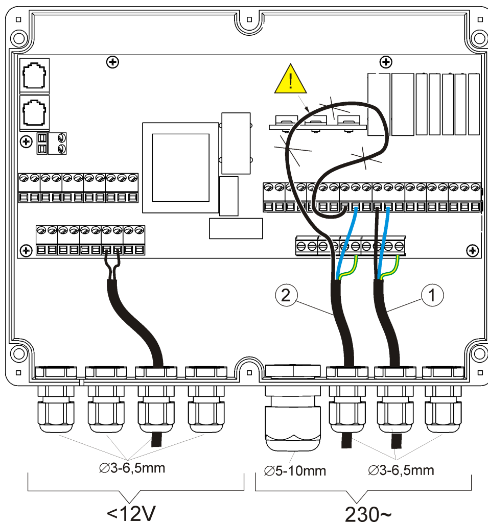
Рис. 21 Подключение проводов, где 1 – правильно подключенный провод, 2 - неправильно подключенный провод (не допускается сматывание лишних проводов внутри устройства).
