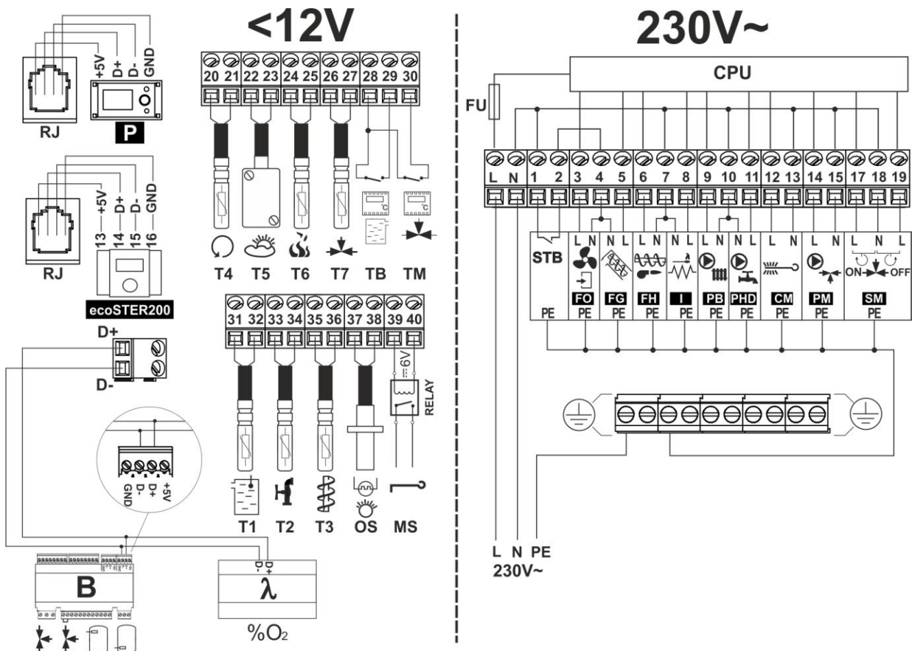
Рис. 22 Схема электрических соединений регулятора , где: T1 – датчик температуры котла СТ4, T2 – датчик температуры горячего водоснабжения СТ4, T3 – датчик температуры подачи, OS – оптический датчик пламени, AL/RB – выход напряжения для сигналов тревоги или управления резервным котлом, RELAY – передатчик, T5 – погодный датчик температуры СТ4-P, T6 – датчик температуры продуктов сгорания СТ2S, T7 – датчик температуры смесителя, TB – вход комнатного термостата котла, TM – вход комнатного термостата смесителя, P – панель управления, ecoSTER – комнатная панель с функцией комнатного термостата (заменяет TB или TM), D-D+ – разъём для дополнительных модулей, B – модуль B расширяет эксплуатацию двух дополнительных контуров смесителей и эксплуатацию теплового буфера, MX.03 – дополнительный модуль расширяет эксплуатацию двух дополнительных смесителей и циркуляционного насоса, λ – модуль зонда Лямбда, L N PE – сетевое напряжение 230V~, FU – сетевой предохранитель, STB – вход ограничителя температуры безопасности, FO – вентилятор наддува горелки, FG – главная подача, I – авторозжиг, PB – Насос котла или буфера, PHD – насос горячего водоснабжения, MP – вытяжной вентилятор котла, PM – двигатель механизма кочерги, SM – привод смесителя, CPU – управление.
