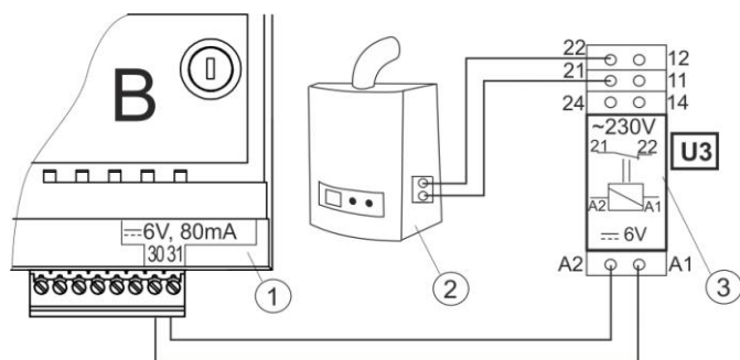
Рис. 24 Пример схемы системы для подключения резервного котла к регулятору Ecomax 800, где: 1 - регулятор ecoMAX700, 2 - резервный котел (газовый или масляный), 3 - Модуль U3, состоящий из реле RM 84-2012-35-1006 и подставки GZT80 RELPOL
