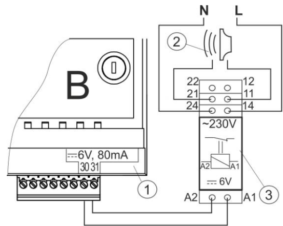
Рис. 28 Подключение внешнего сигнального устройства, где: 1- регулятор , 2 –внешнее сигнальное устройство, 3 – передатчик.
