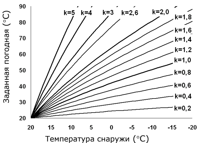
Рис. 9 Кривые нагрева.
