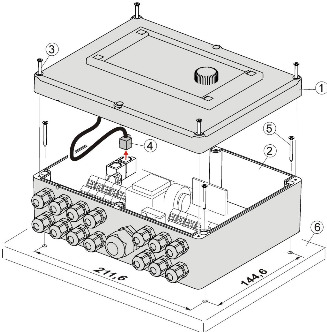
Рис. 20 Установка регулятора на монтажной поверхности, где: 1 – крышка, 2 – подставка, 3 – шуруп крышки, 4 – штекер, 5 – шуруп, крепящий к монтажной поверхности, 6 – монтажная поверхность.
