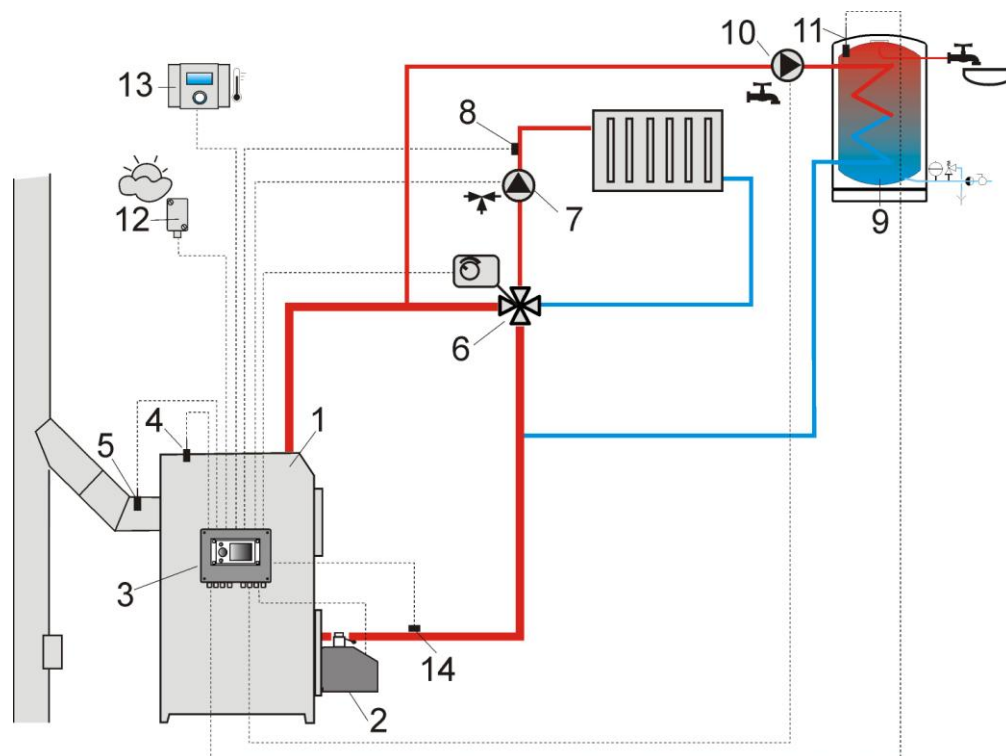
Рис. 17 Схема с четырехходовым клапаном, управляющим контуром центрального отопления 3 , где: 1 – котёл, 2 – горелка, 3 – регулятор, 4 – датчик температуры котла СТ4, 5 – датчик температуры продуктов сгорания СТ2S (только просмотр температуры), 6 – привод четырехходового клапана, 7 – насос контура смесителя, 8 – датчик температуры контура смесителя, 9 – резервуар горячего водоснабжения, 10 – насос горячего водоснабжения, 11 – датчик горячего водоснабжения, 12 – погодный датчик температуры СТ4-Р, 13 – комнатная панель ecoSTER или стандартный комнатный термостат, 14 – датчик температуры возврата (не является необходимым для работы системы).
