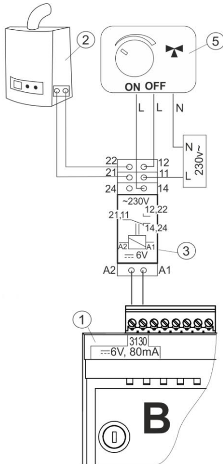
Рис. 26 8 Схема электрических соединений управления переключающим клапаном резервного котла, где: 1 – регулятор, 2 – Резервный котел, 3 – передатчик, 5 – привод переключающего клапана (с конечными выключателями), Внимание: зажимы 22,21,24 должны быть гальванически отделены от зажимов 12,11,14.
