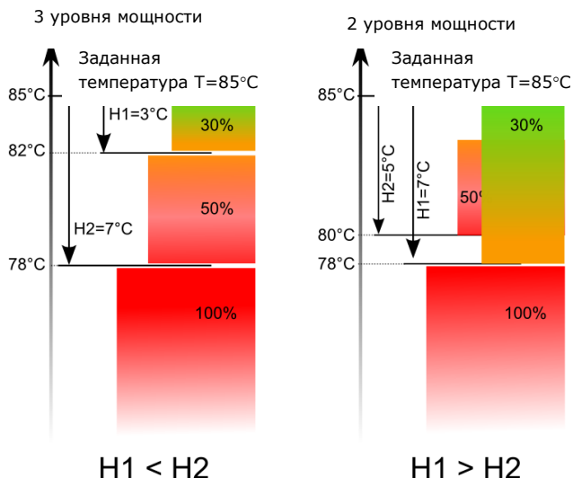
Рис. 8 Гистерезисы H1 и H2 регулирования мощности
