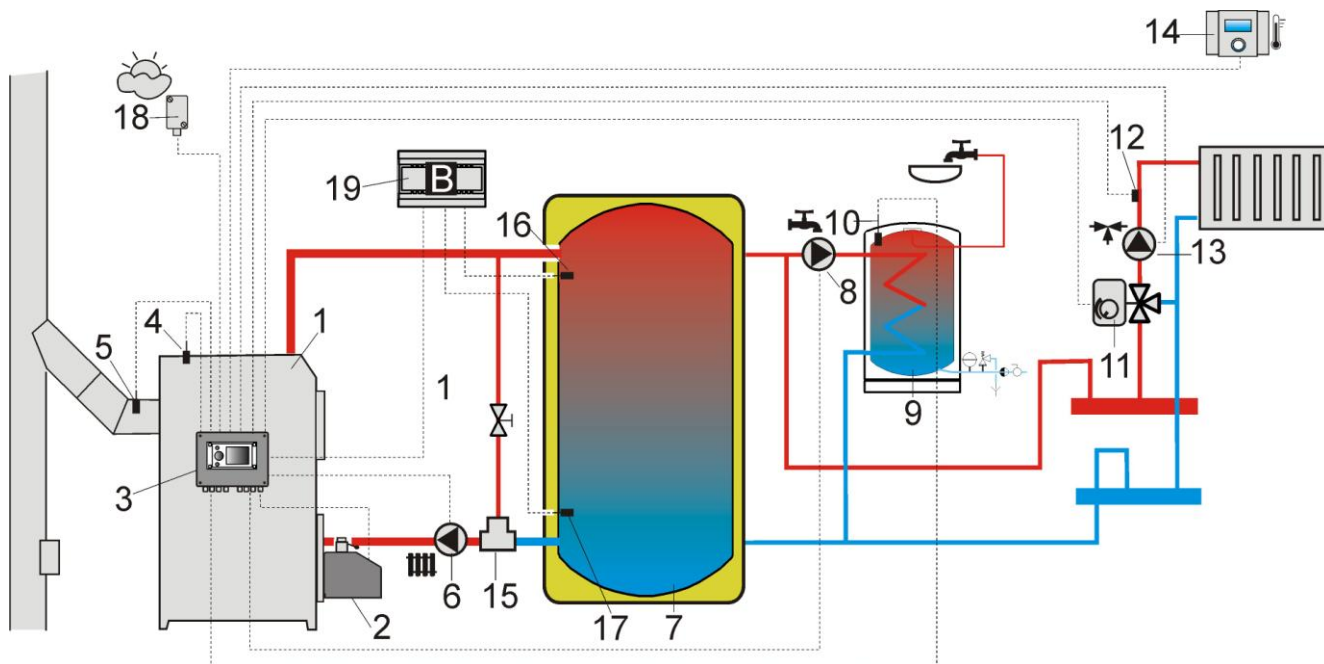
Рис. 18 Схема с тепловым буфером 4 , где: 1 – котёл, 2 – горелка, 3 – регулятор, 4 – датчик температуры котла, 5 – датчик температуры продуктов сгорания (только просмотр температуры), 6 – Насос котла, 7 – тепловой буфер, 8 – насос горячего водоснабжения, 9 – резервуар горячего водоснабжения, 10 – датчик температуры горячего водоснабжения, 11 – привод смесительного крана, 12 – датчик температуры контура смесителя, 13 – насос смесителя, 14 – комнатная панель ecoSTER с функцией комнатного термостата, 15 – термостатический трехходовой клапан для защиты возврата, 16 – датчик температуры буфера верхний, 17 – датчик температуры буфера нижний, 18 – погодный датчик температуры, 19 – дополнительный модуль В.
