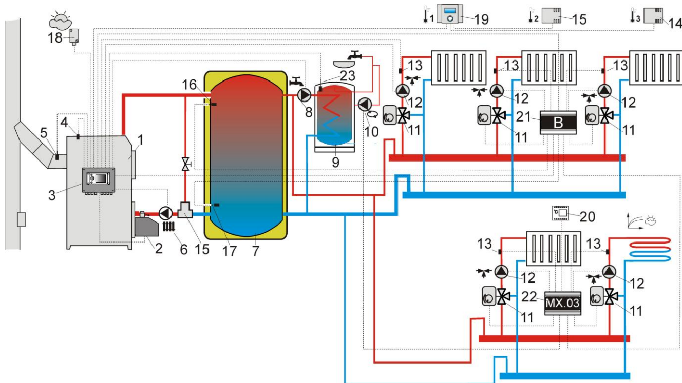
Рис. 19 Схема с тепловым буфером и с 5 смесительными нагревательными контурами 5 , где: 1 – котёл, 2 – горелка, 3 – регулятор, 4 – датчик температуры котла СТ4, 5 – датчик температуры продуктов сгорания СТ2S, 6 – Насос котла, 7 – тепловой буфер, 8 – насос горячего водоснабжения, 9 – резервуар горячего водоснабжения, 10 – циркуляционный насос, 11 – трехходовой клапан с приводом, 12 – насос контура смесителя, 13 – датчик температуры контура смесителя СТ4, 14 – комнатная панель ecoSTER, 15 – комнатная панель ecoSTER, 16 – верхний датчик температуры буфера СТ4, 17 – нижний датчик температуры буфера СТ4, 18 – погодный датчик температуры СТ4-Р, 19 – комнатная панель ecoSTER, 20 – стандартный комнатный термостат (замыкательно-размыкательный), 21 – дополнительный модуль В, 22 – дополнительный модуль МХ.03, 23 – датчик температуры горячего водоснабжения.
