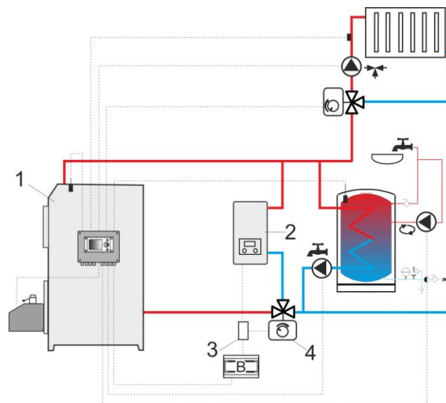
Рис. 25 7 Гидравлическая схема с резервным котлом в закрытом контуре, где: 1 - регулятор, 2 - Резервный котел, 3 - передатчик (Рис. 27), 4 - переключающий клапан (с конечными выключателями).
