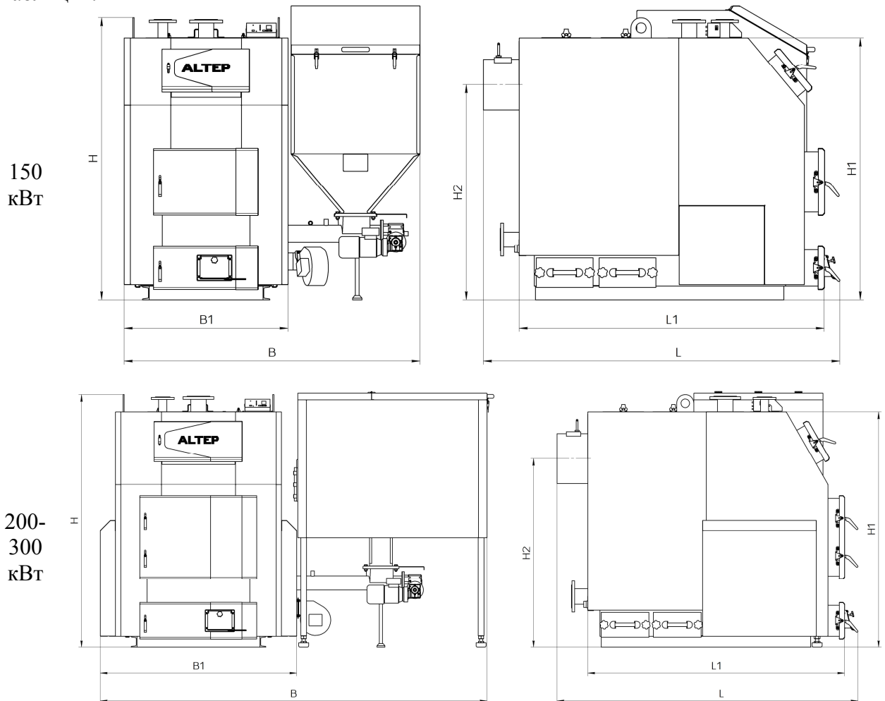
Рисунок 1 – Габаритне креслення котла типу КТ-3Е-SH
