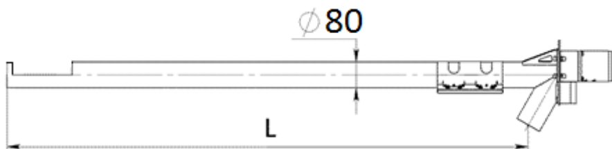
Рис.2 Геометрия комплектного шнека KVIТ Optima
